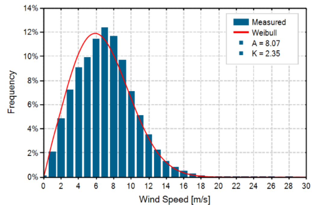
Figure 6 : Courbe de Weibull (source : VALECO, 2020)
